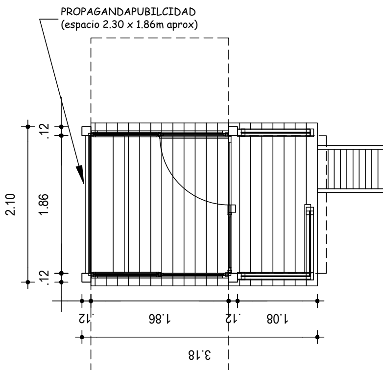
PLANTA esc 1:50
